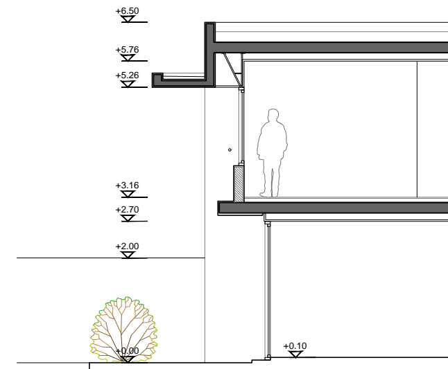
DETALLE 1
