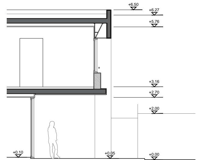
DETALLE 1
