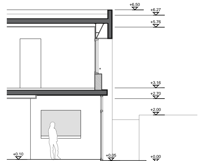
DETALLE 2
