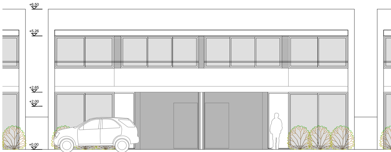
FACHADA FRONTAL
