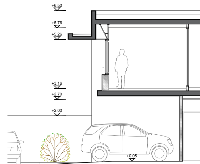
DETALLE 2
